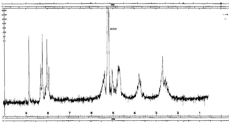
Fig. 2. ^1\text{H} -NMR.-Spektrum von N (10)-Nitroso-leucovorin (VI) in 0,1N NaOD
