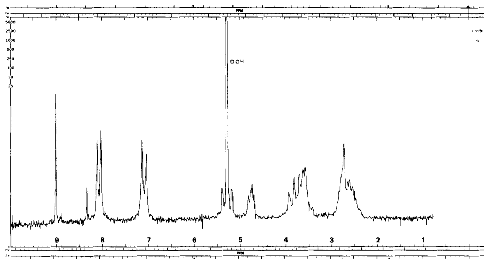
Fig. 1. ^1\text{H} -NMR.-Spektrum von Leucovorin (II) in 0,1N NaOD
